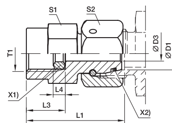
X1) Kroužek DKL s těsnící hranou X2) O-kroužek OR
