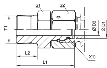
X1) O-kroužek OR
