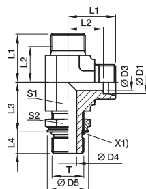
X1) O-kroužek OR
