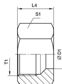
Převlečná matice M
