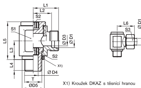
X1) Kroužek DKAZ s těsnící hranou
