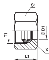
X1) Opěrný kroužek
